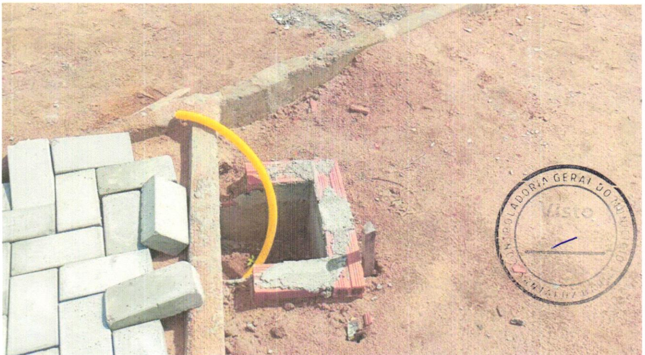
FOTO 14 - Caixa de passagem em alvenaria de tijolos maciços esp. = 0,12m, dim. int. = 0,30 x 0,30 x 0,30m
